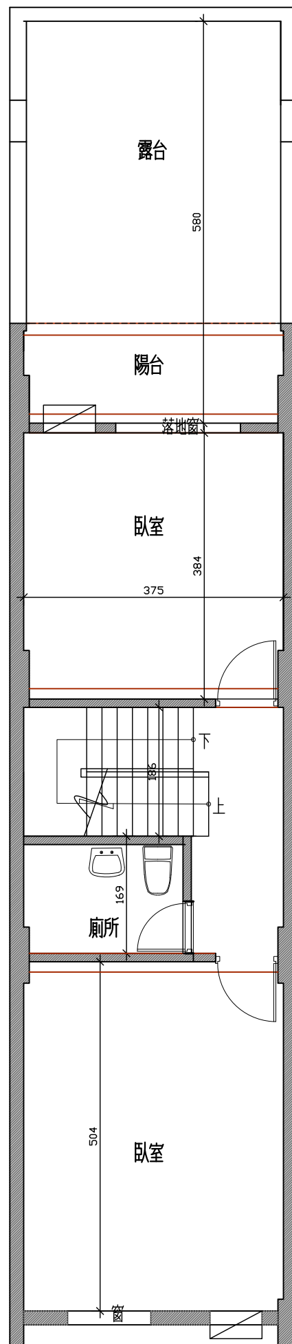
四樓平面圖
