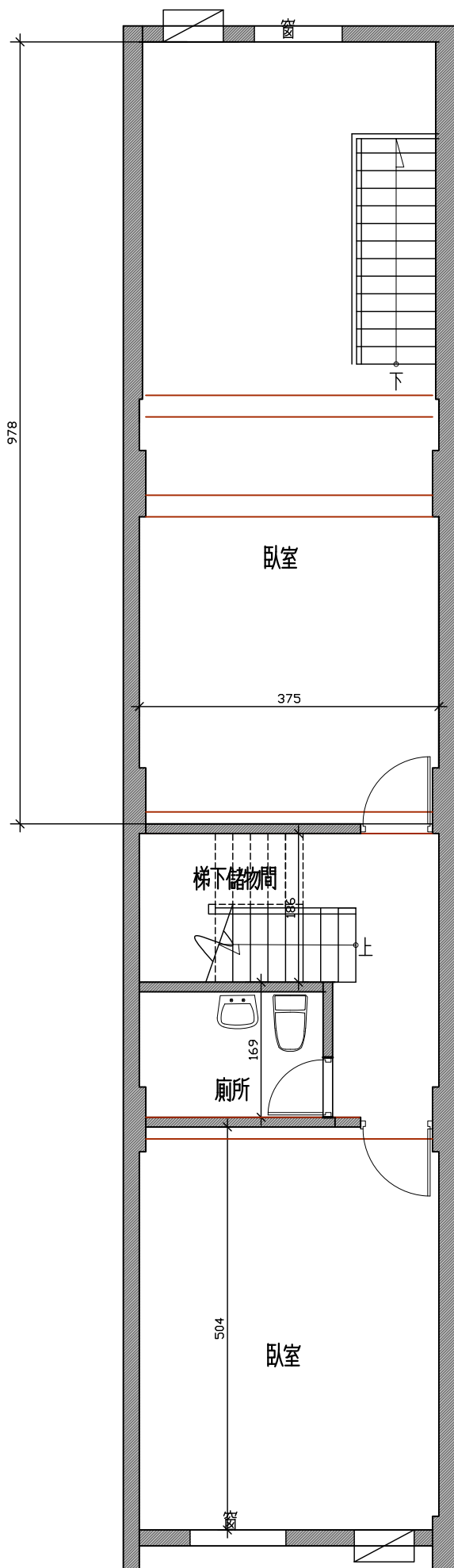
三樓平面圖
