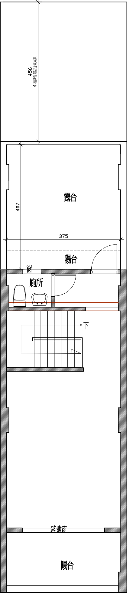
五樓平面圖
